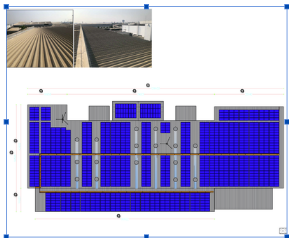
บริษัท นิตโต เดนโกะ แมททีเรียล (ประเทศไทย) จำกัด 999.57 kWp
