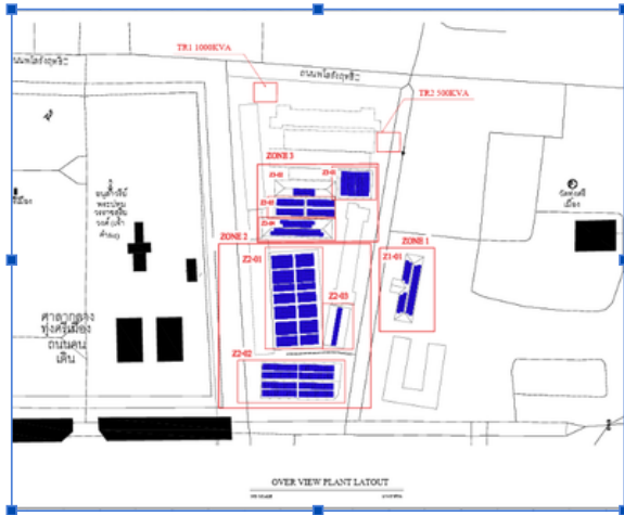
โรงเรียนอนุบาลอุบลราชธานี 999.18 kWp
