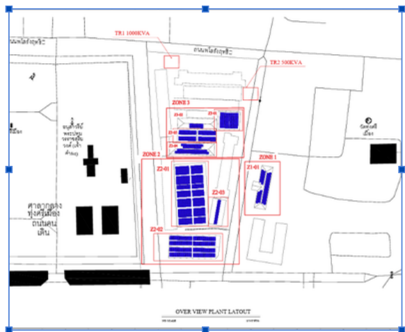
โรงเรียนโพธิ์ไทรพิทยาคาร อุบลราชธานี 127.8 kWp
