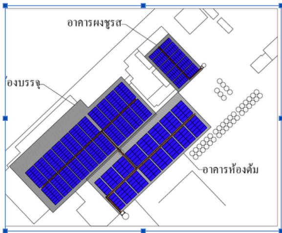
บจก. เจริญมงคล ฟู้ดส์ แอนด์ เบฟเวอเรจ 393.45 kWp
